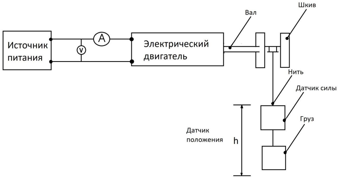
Рис.2 Схема установки
