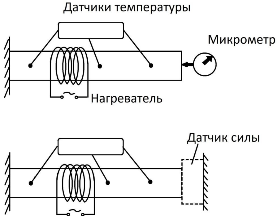
Рис.1 Схема установки
